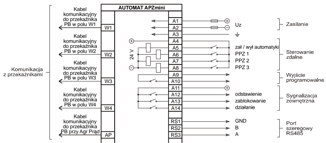
Rys. 6. Schemat podłączeń zewnętrznych automatu APZmini.
