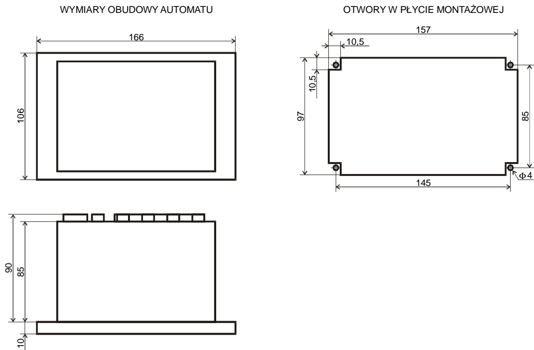
Rys. 2. Obudowa automatu APZmini.
