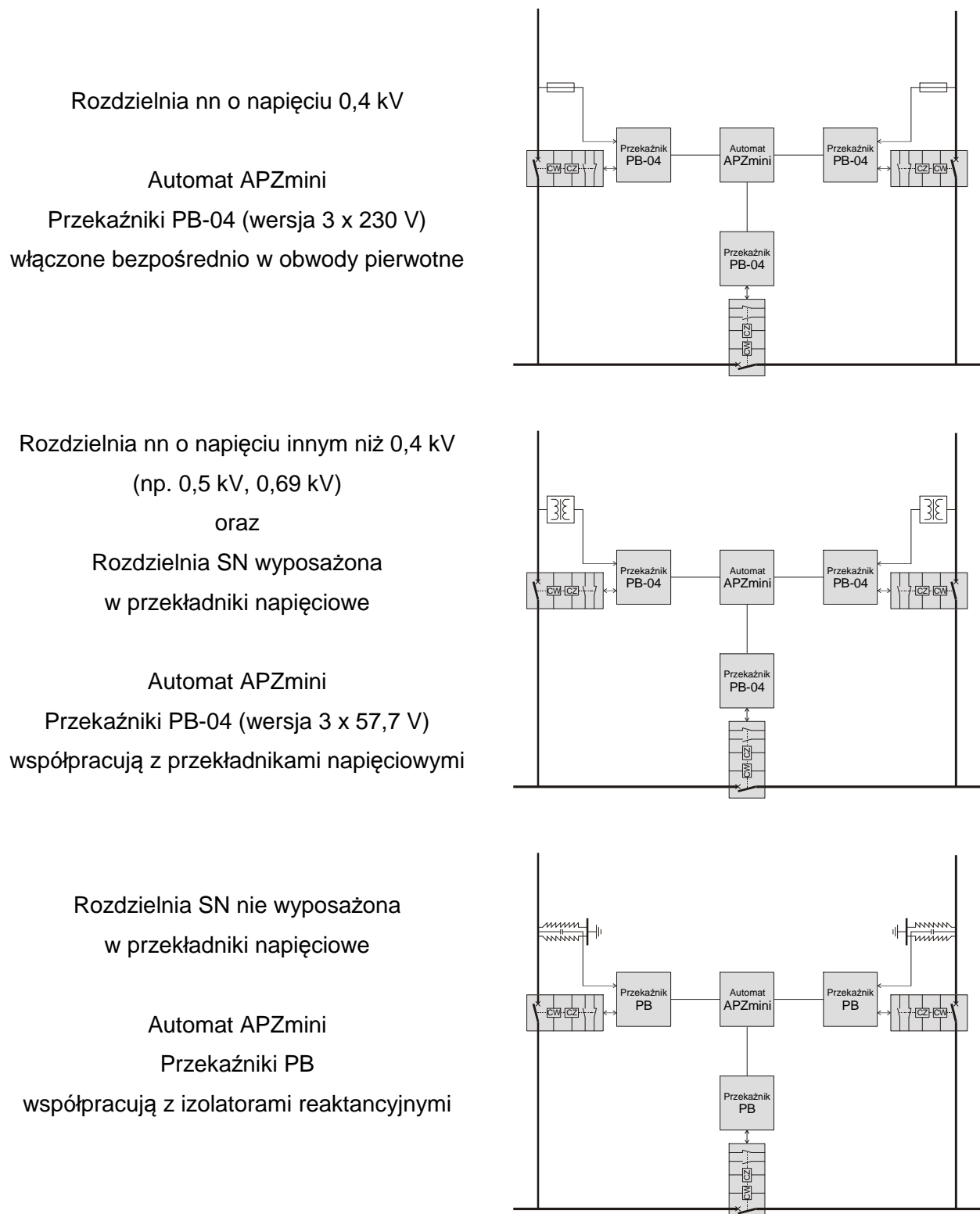
Rys. 1. Przykładowa struktura układu automatyki przełączania zasilania dla rozdzielni pracujących w układzie rezerwy ukrytej.
