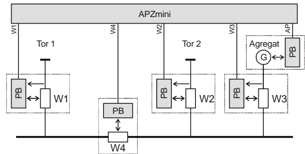
Rys. 5. Rozmieszczenie urządzeń automatyki przełączania zasilania oraz połączenia komunikacyjne pomiędzy przekaźnikami PB (lub PB-04) a automatem.
